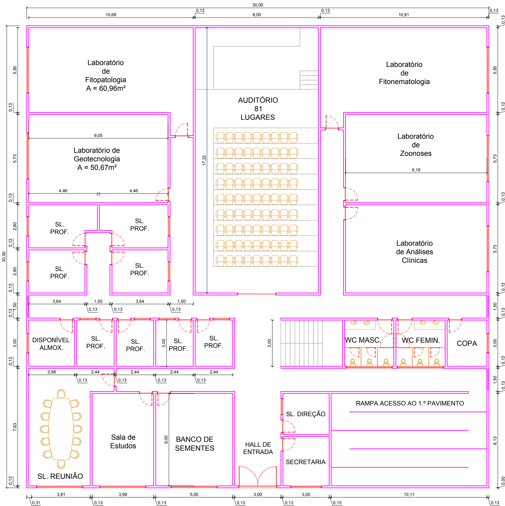
PLANTA BAIXA - PAVIMENTO TÉRREO TIPOLOGIA - EDUCACIONAL ESCALA 1:100 ÁREA DO PAVIMENTO: 900,00m²
