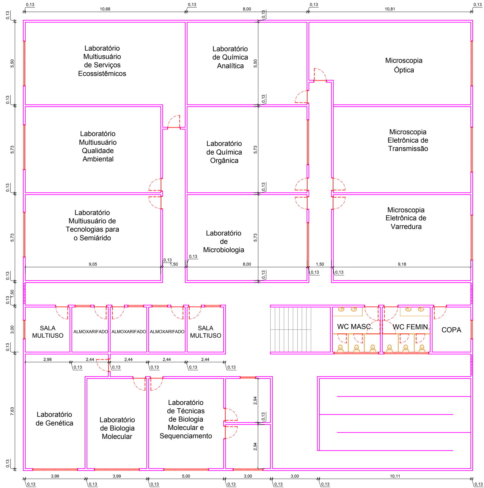
PLANTA BAIXA - PAVIMENTO SUPERIOR
